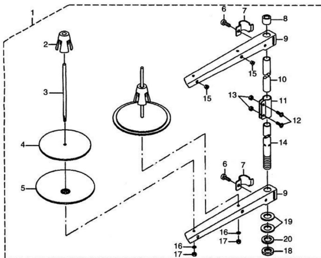
F 12. COMPONENTES DEL SOPORTE DE HILOS
